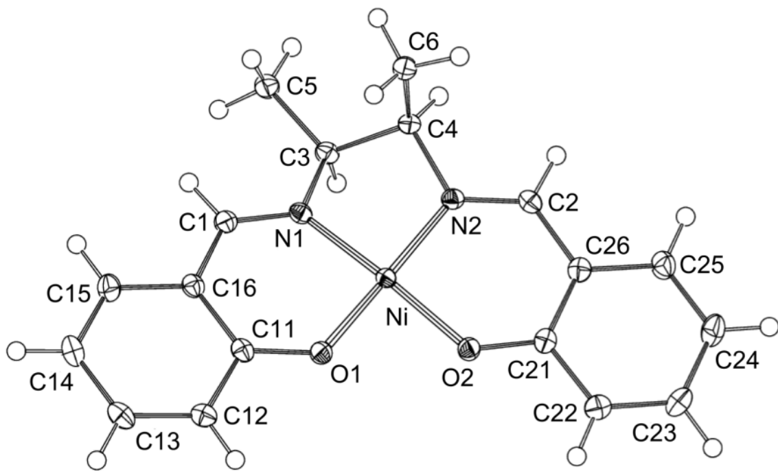
monomer
