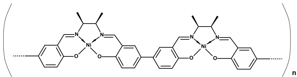
4 polimer
